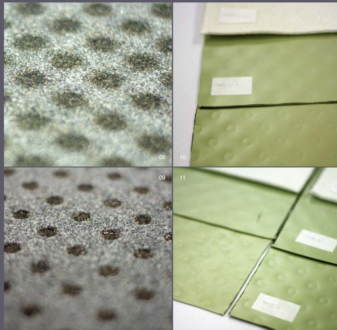
08, 09 | Vliv použití geotextilie na otláčení asfaltového pásu na tuhém podkladu
