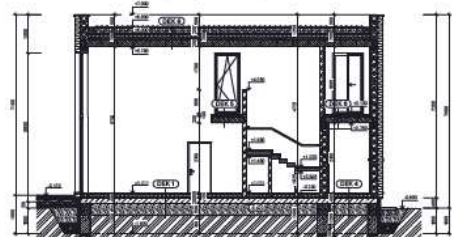
REZ OBJEKTEM B - B'
