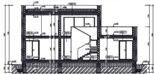
REZ OBJEKTEM B - B'
