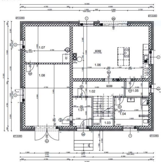
PŮDORYS 1.NP
